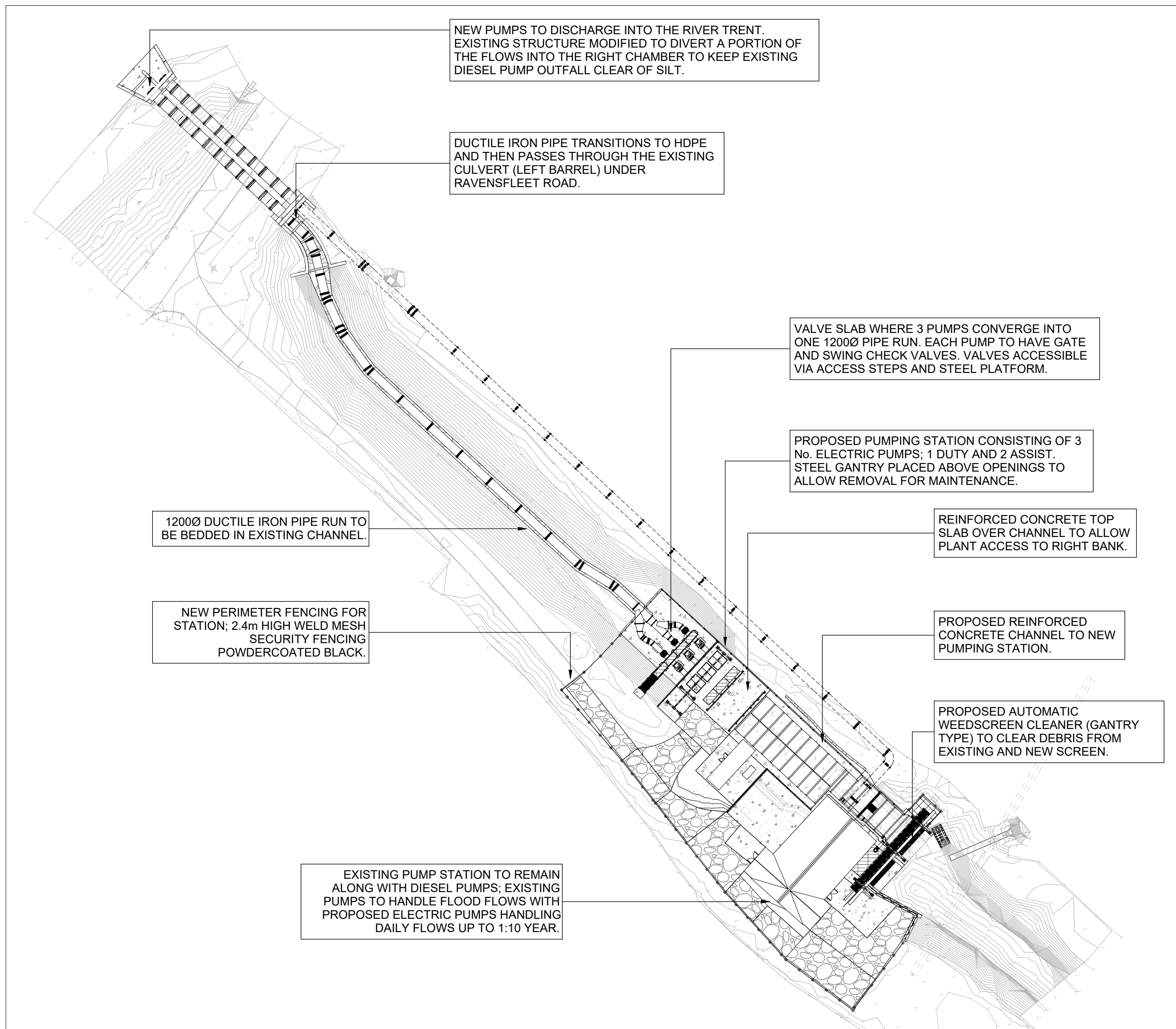
SITE OVERVIEW - PLAN SCALE 1 : 500
