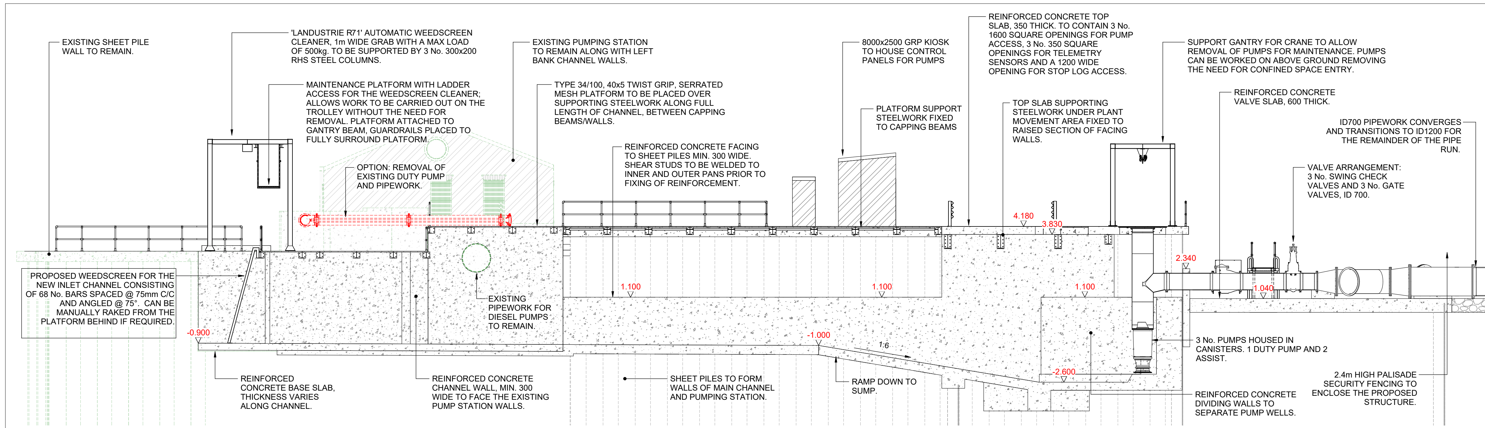
SITE OVERVIEW - SECTION 1-1 SCALE 1 : 100
